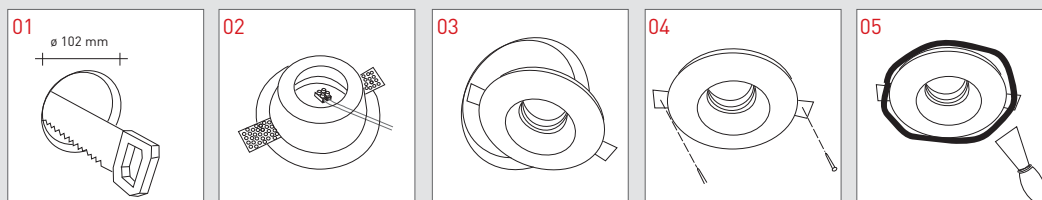
Schema di montaggio Assembly diagram Montageplan Esquema de montaje Схема монтажа
