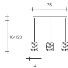
1497.31 _ 3x60W _ G9
