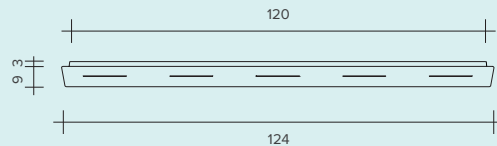
G9 5X max 28W - 230V
