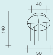
G9 5X max 28W - 230V
