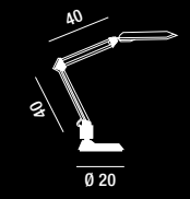
4026 A Lampada da tavolo orientabile in plastica colore argento Adjustable plastic silver table lamp
