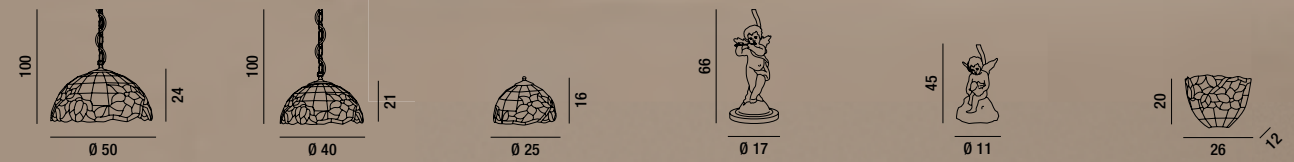
T614 S Sospensione Tiffany con catena Tiffany hanging lamp with chain T616 S Sospensione Tiffany con catena Tiffany hanging lamp with chain B616 Lampada da tavolo in resina e zama senza paralume Zama resin table lamp without shade B618 Lampada da tavolo in resina e zama senza paralume Zama resin table lamp without shade T618 A Applique Tiffany Tiffany wall lamp 3XE27 MAX 60W H. REGOLABILE 1XE27 MAX 100W H. REGOLABILE 1XE27 MAX 60W 1XE27 MAX 60W 1XE27 MAX 60W
