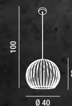
5858 B Sospensione acrilico bianco Acrylic white hanging lamp
