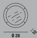
5646 Applique alluminio per esterni colore grafite con diffusore in acrilico Outdoor graphite aluminium wall lamp with acrylic diffuser
