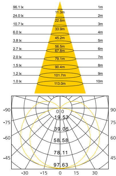
LD2BAR102
