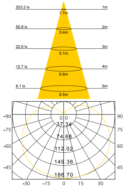
LD2BAR202
