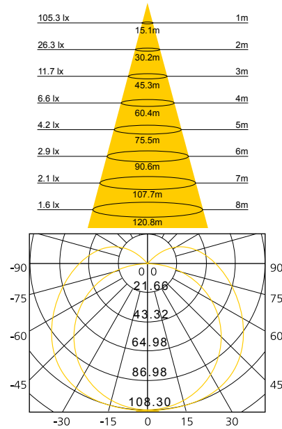
LD2BAR103
