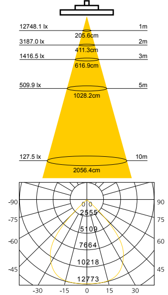
LD1HB220G - 120°
