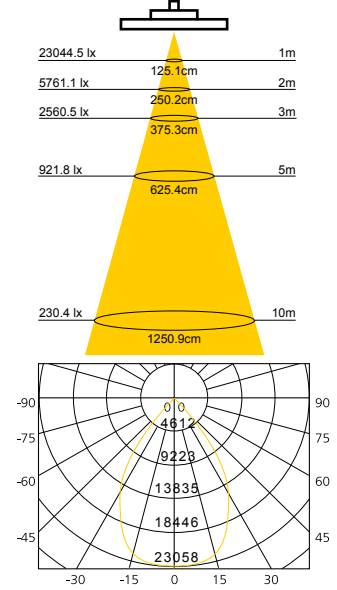
LD1HB220G - 90°
